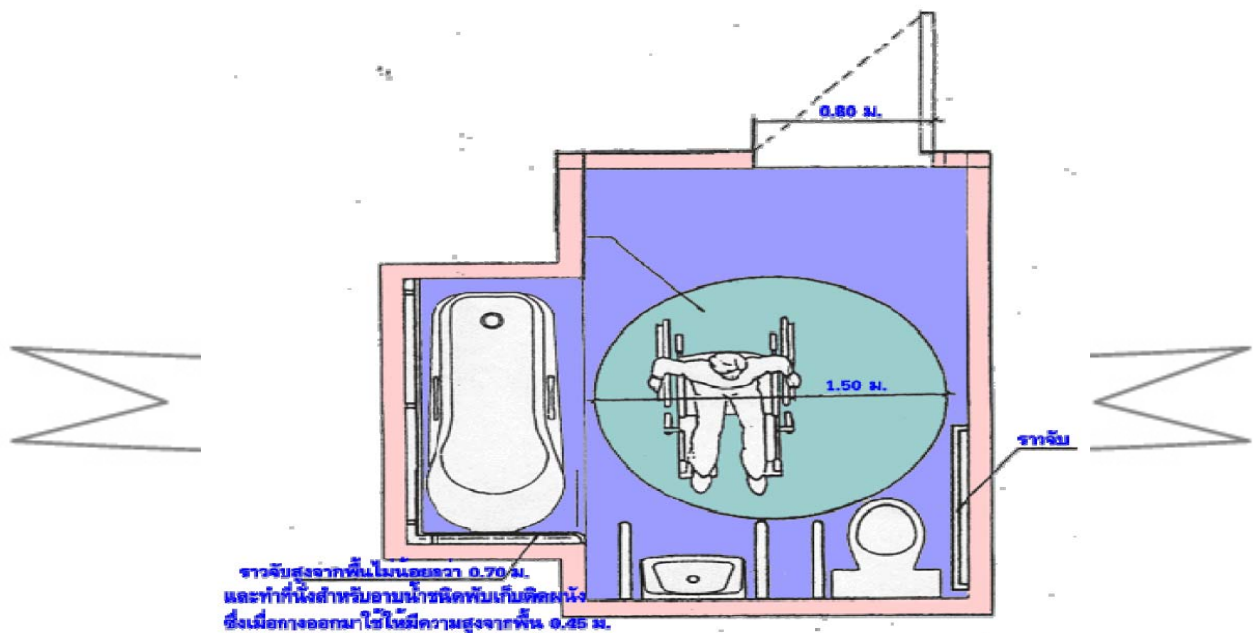
ภาพที่ 36 รูปประตูและห้องน้ำคนพิการ หมายเลข 10
