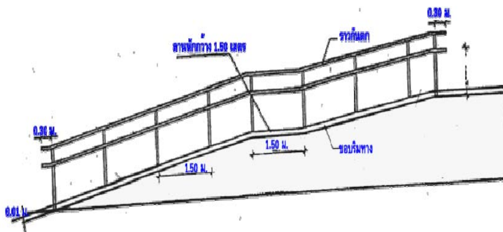
ภาพที่ 29 รูปทางลาดพร้อมราวจับ หมายเลข 3
