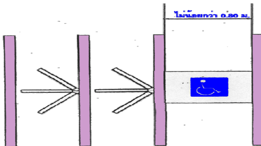
ภาพที่ 41 รูปทางเข้าออกที่มีเครื่องกั้นหรือช่องรับบริการ หมายเลข 14 ที่มา : ธนายุทธ ชนธิต,ประฤดา สุริยันต์ และยูวดี อิศราชาติ., “รายงานการวิจัย เรื่องสิ่งอำนวยความสะดวกสำหรับคนพิการและเพื่อทุกคนในสังคม,” กระทรวงการพัฒนาสังคมและความมั่นคงของมนุษย์ 2549 : 243.
