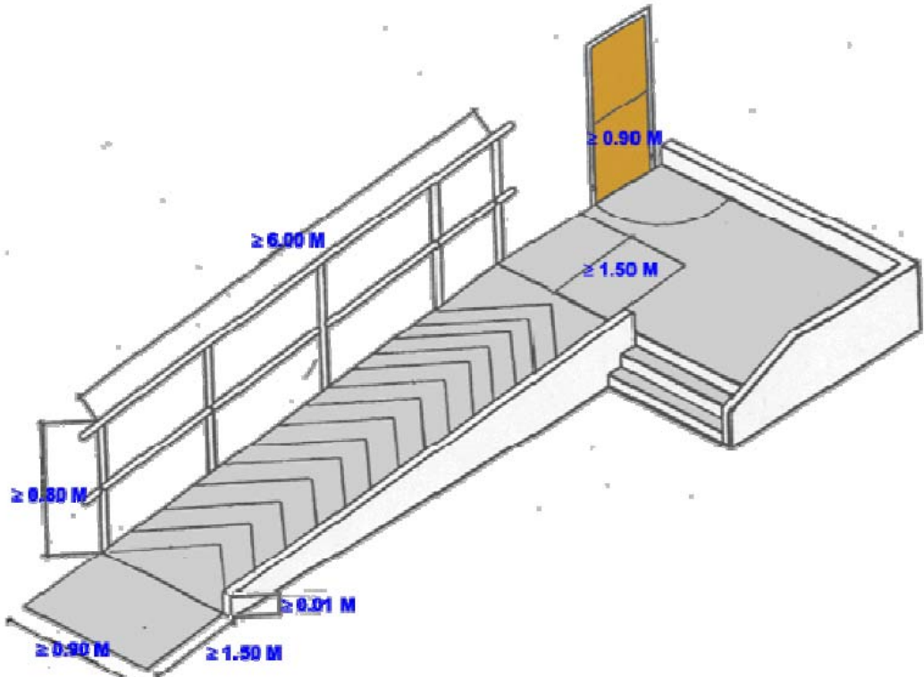
ภาพที่ 27 รูปทางลาด หมายเลข 1
