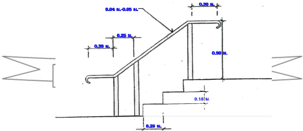
ภาพที่ 32 รูปราวจับบันได หมายเลข 6 ที่มา : ธนายุทธ ชนธิต, ประฤดา สุริยพันธ์ และยูวดี ถิรธราดล., “รายงานการวิจัย เรื่องสิ่งอำนวยความสะดวกสำหรับคนพิการและเพื่อทุกคนในสังคม,” กระทรวงการพัฒนาสังคมและความมั่นคงของมนุษย์ 2549 : 236.
