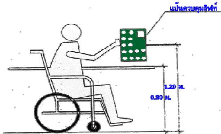
ภาพที่ 35 รูปปุ่มบังคับลิฟท์ หมายเลข 9
