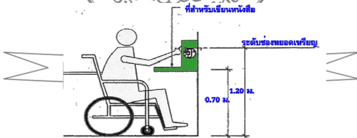
ภาพที่ 42 รูปที่ตั้งโทรศัพท์สาธารณะ หมายเลข 15 ที่มา : ธนายุทธ ชนธิต,ประฤดา สุริยันต์ และยูวดี อิศราชาติ., “รายงานการวิจัย เรื่องสิ่งอำนวยความสะดวกสำหรับคนพิการและเพื่อทุกคนในสังคม,” กระทรวงการพัฒนาสังคมและความมั่นคงของมนุษย์ 2549 : 246.
